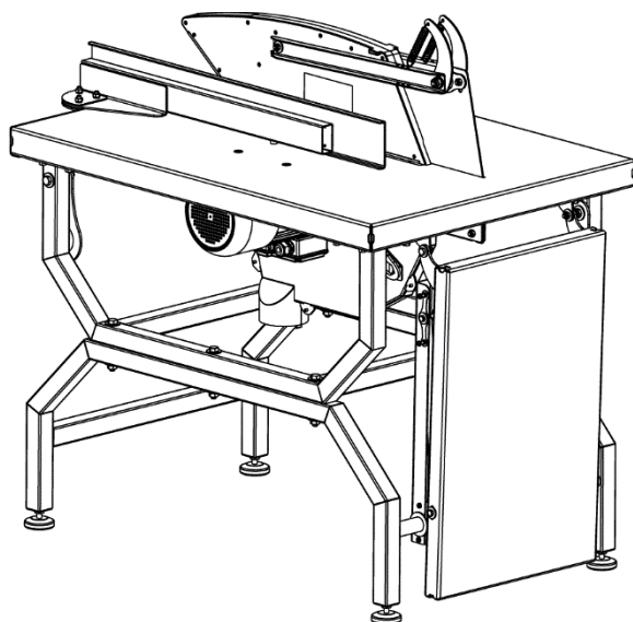
Рисунок 2. Общий вид станка со сложенным дополнительным столом
