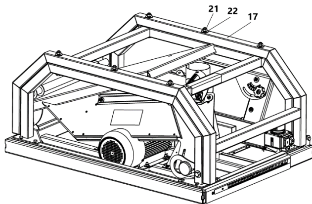
Рисунок 4 Общий вид станка в упаковке 17 – основание, 21 – гайка M10, 22 – болт M10×100
